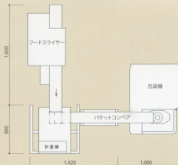
ワンタッチ脱着バケット
